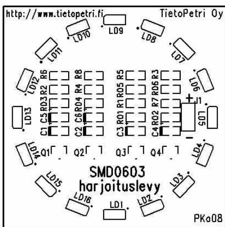
Kuva 5. Piirilevy
