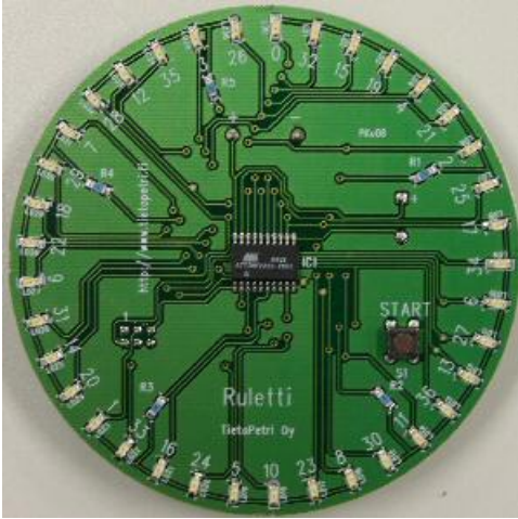
Kuva 1. Kasattu piirilevy
