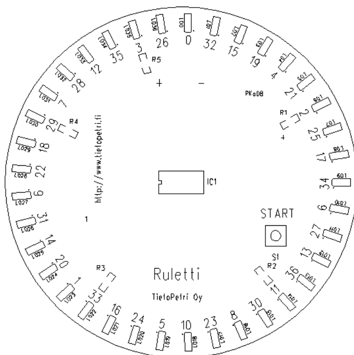
Kuva 5. Piirilevy
