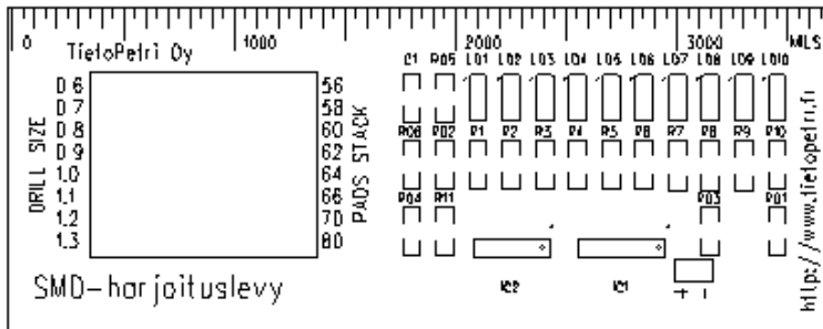
Kuva 5. Piirilevy
