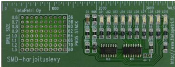
Kuva 1. Kasattu piirilevy
