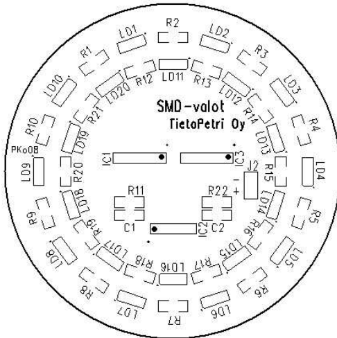
Kuva 5. Piirilevy
